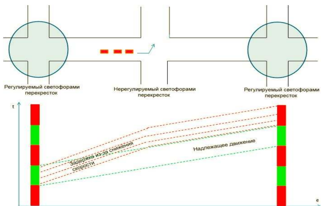
Рисунок 3.4.3 – Схема влияния нерегулируемого пересечения на координированное управление
