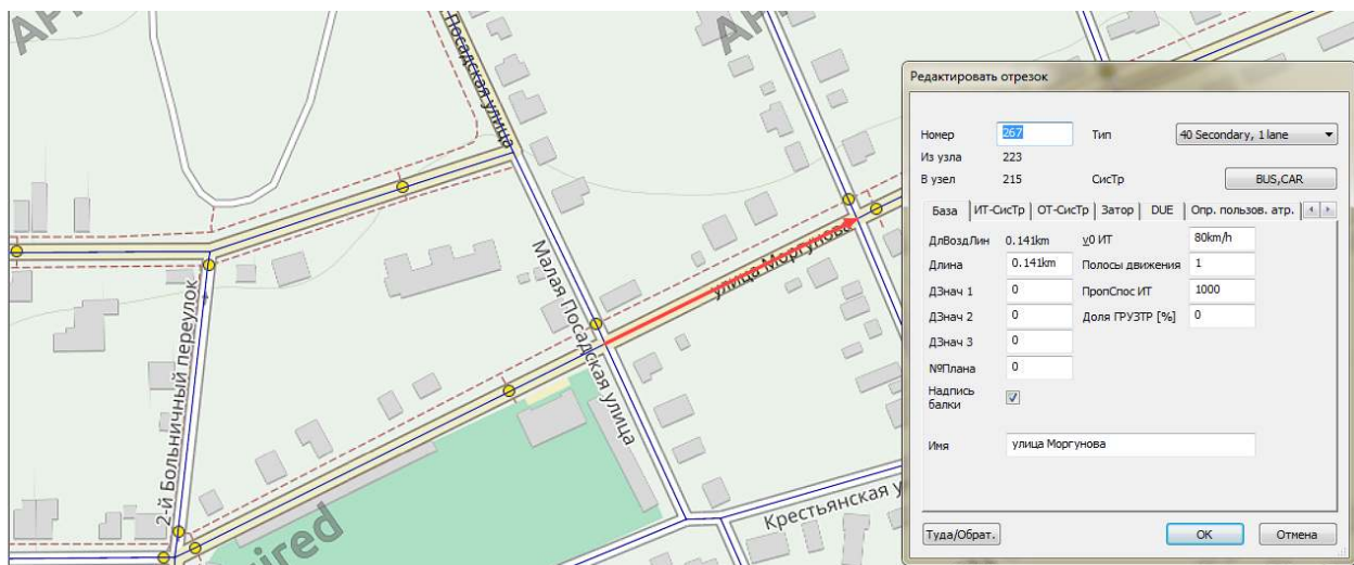
Рисунок 9 – Редактирование отрезка
