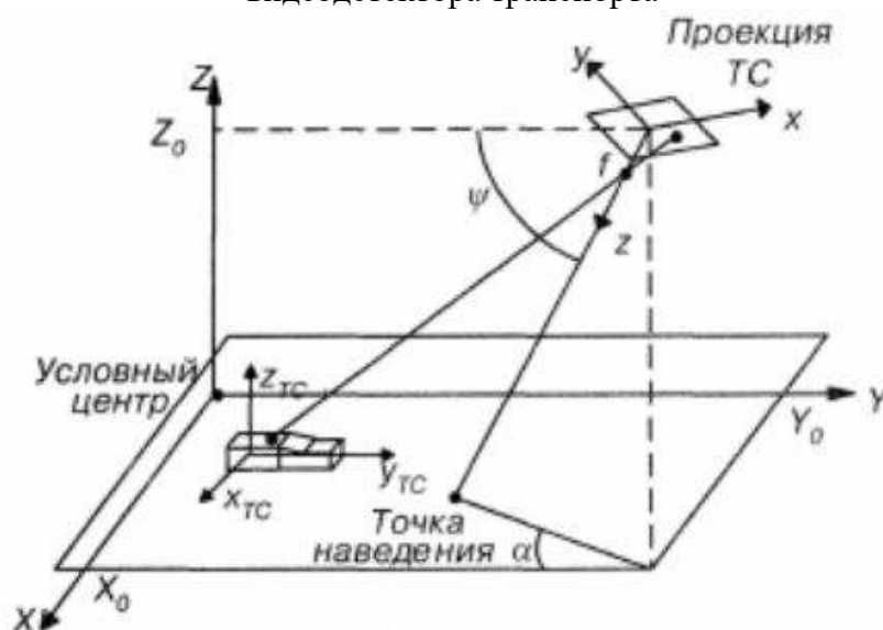
Рисунок 3.12.2 – Общая схема установки детектора транспорта
