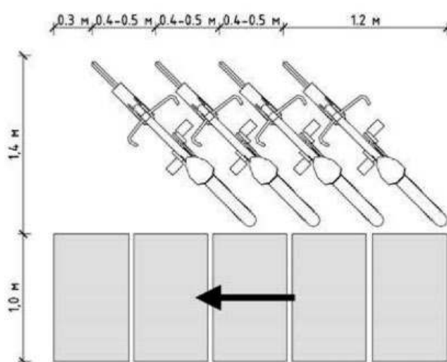
Рисунок 3.5.2 – Диагональное расположение велосипедов
