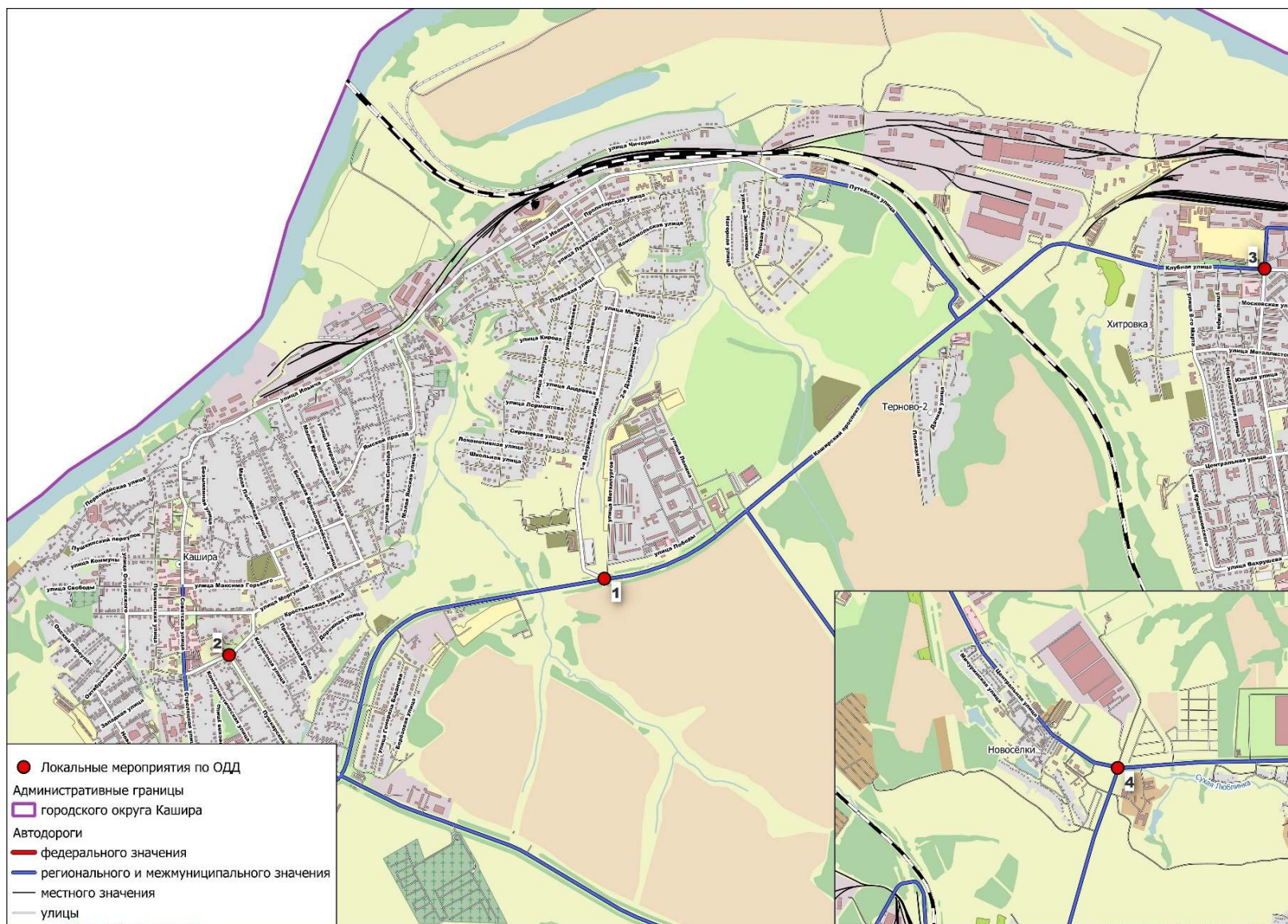
Рисунок 3.2.14 – Схема расположения узлов, на которых предлагаются локальные мероприятия по повышению пропускной способности дорог, формированию кольцевых пересечений и примыканий дорог, реконструкции перекрестков
