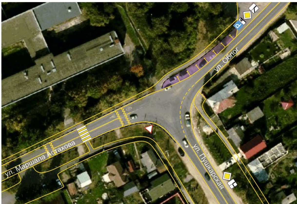
Рисунок 3.2.2 – Схема локальных мероприятий на узле ул. Пушкинская и ул. Маршала Астахова
