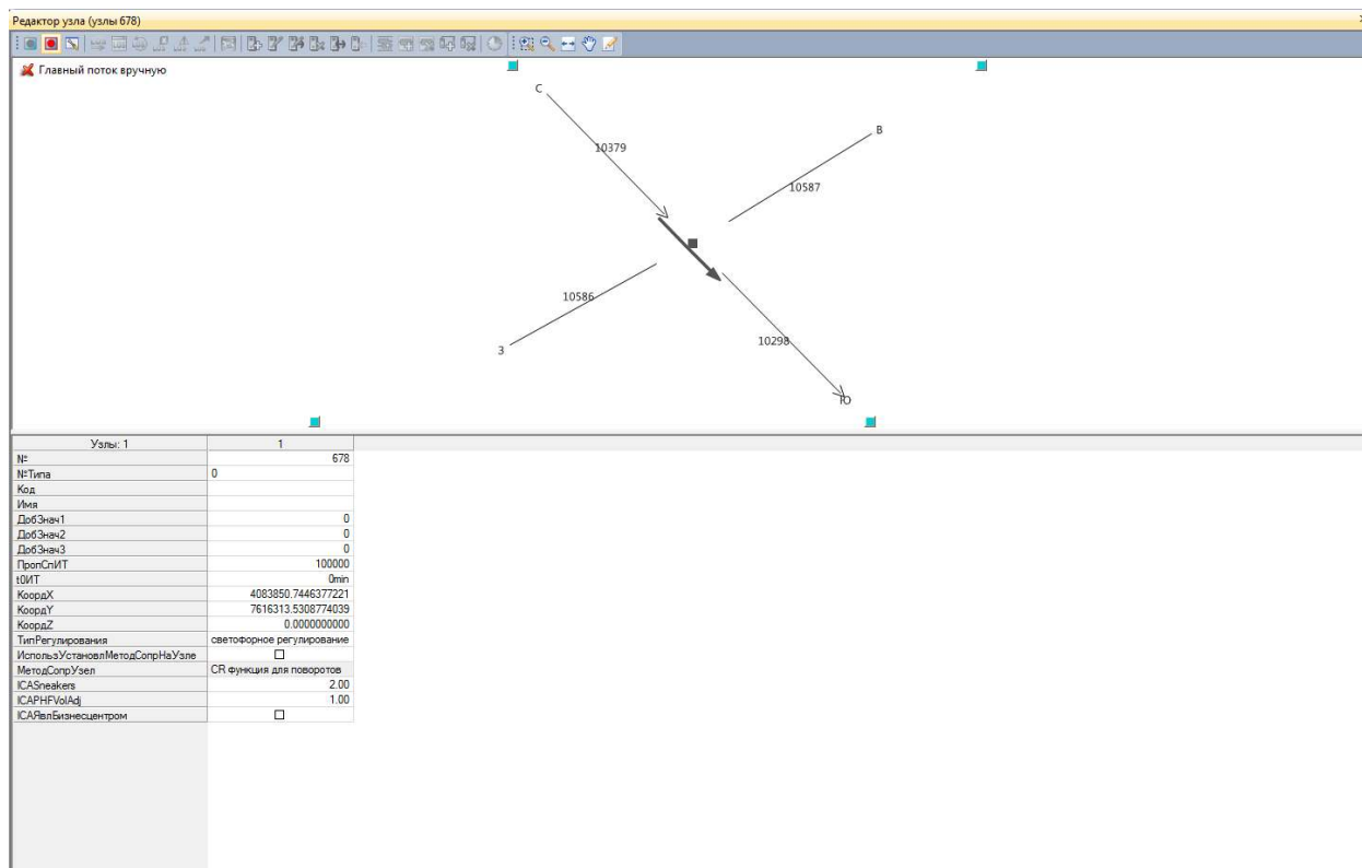
Рисунок 7 – Редактирование узла
